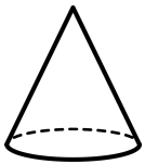
Cone
